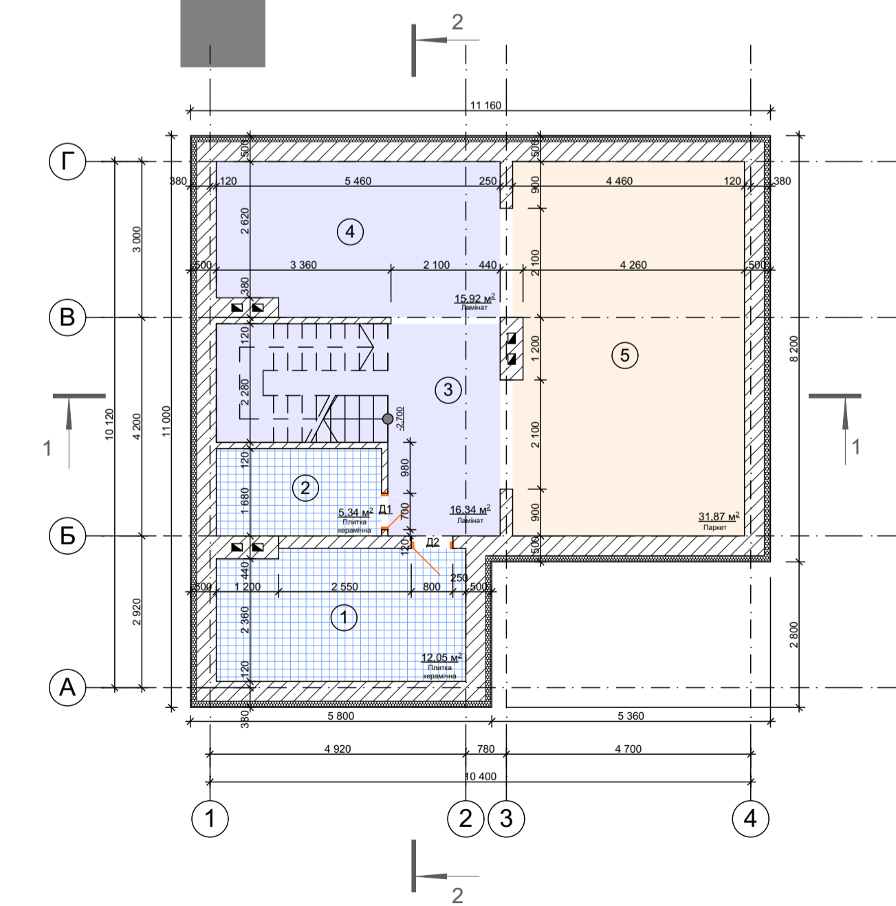
План цокольного поверху М1:100
