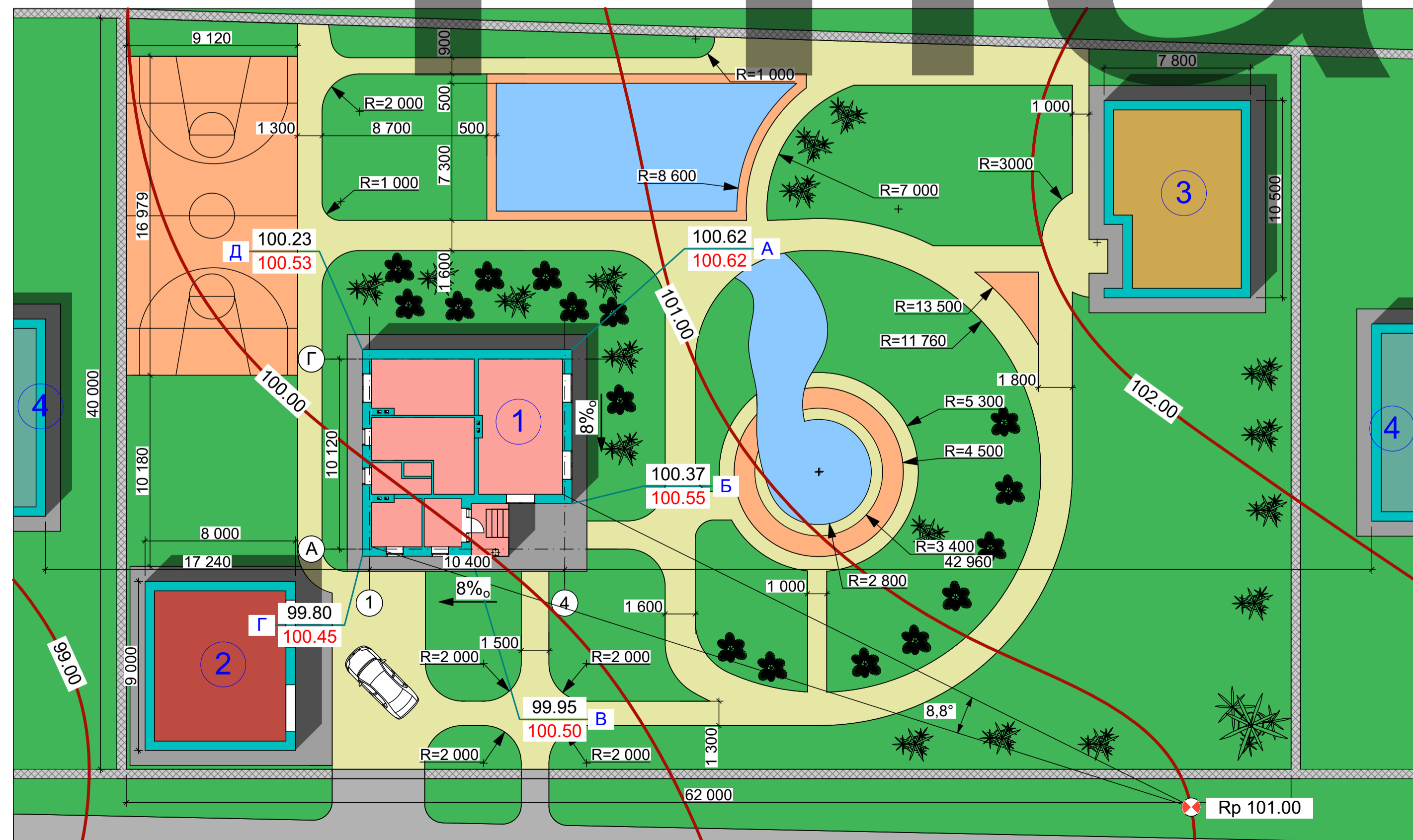
Генеральний план М1:200
