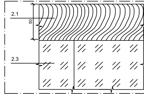
POHĽAD M 1:2
