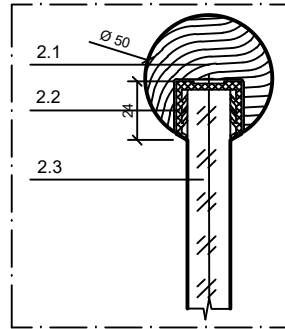
DETAIL 2 M 1:2
