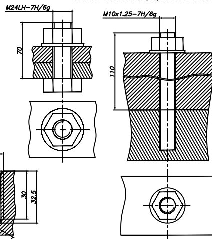
Упрощенные изображения соединений болтом и шпилькой (2-1) ГОСТ 2.315-68
