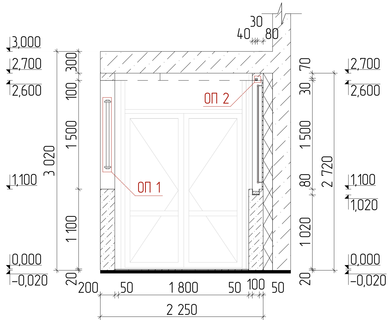
Переріз 1-1 М 1:30
