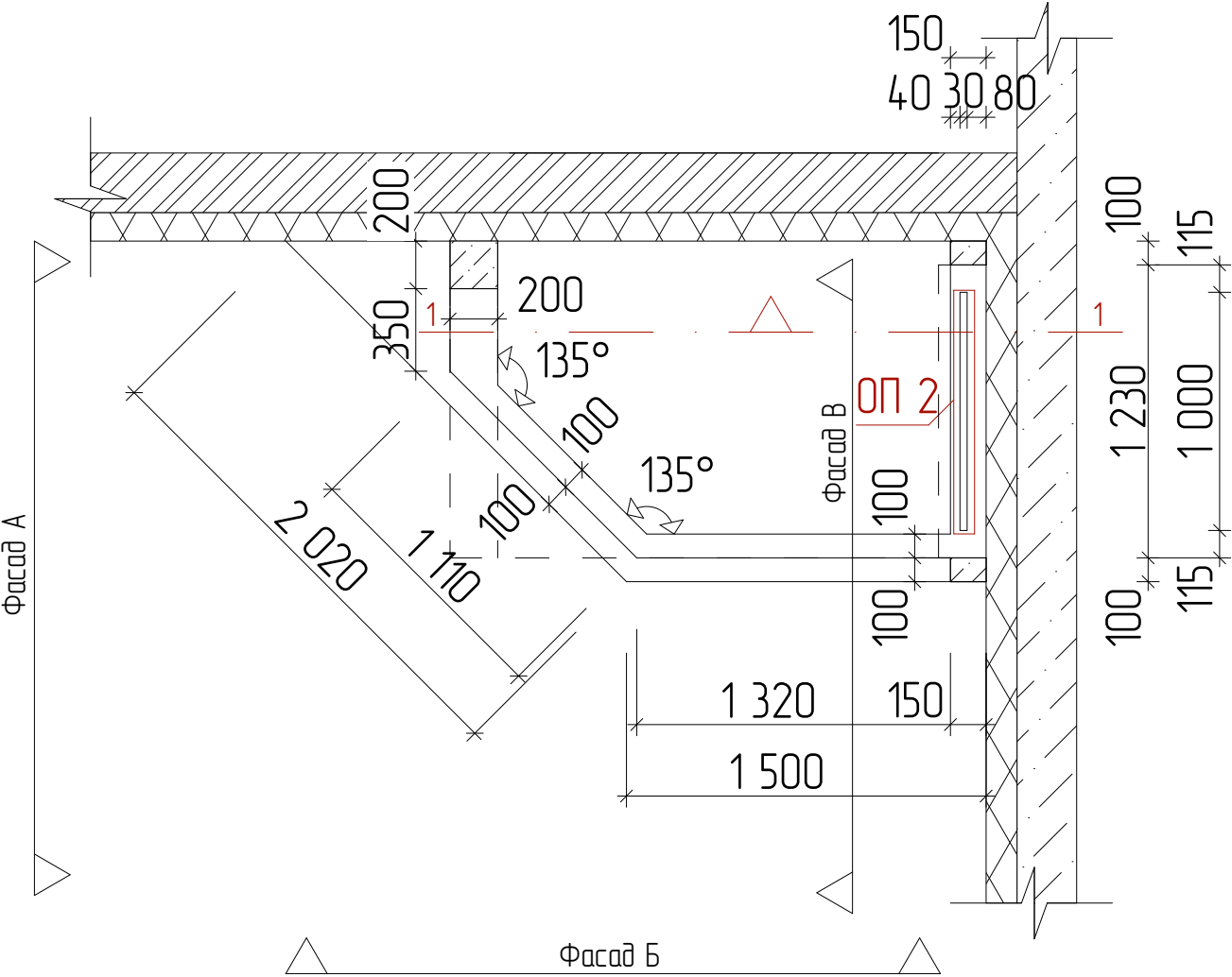
План дашку М 1:30
