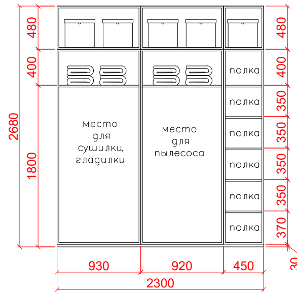
ВНУТРЕННЕЕ НАПОЛНЕНИЕ ШКАФА
